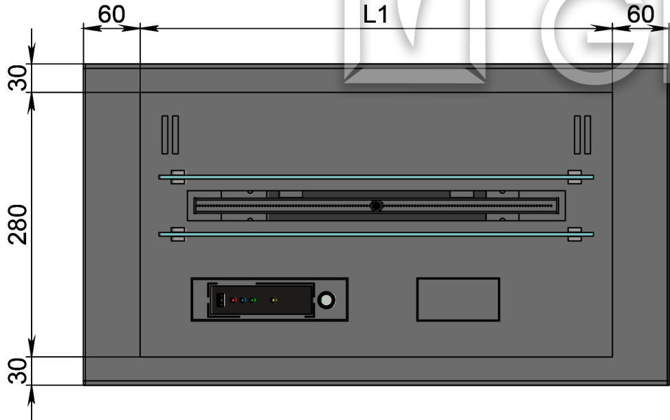
Вид сверху
