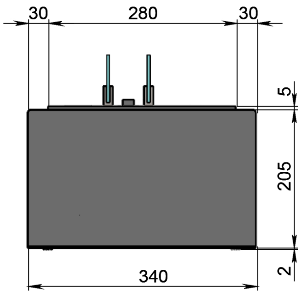
Вид сбоку
