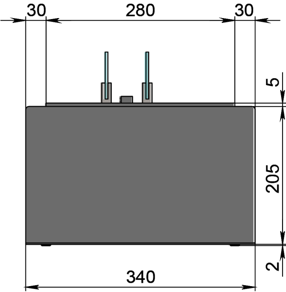
Вид сбоку
