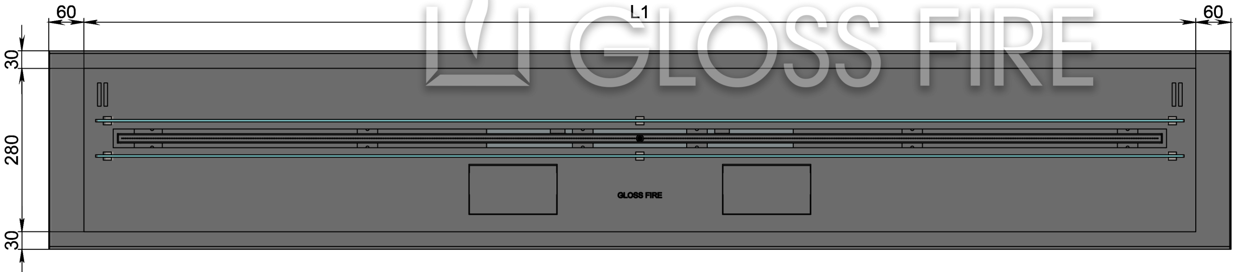
Вид сверху
