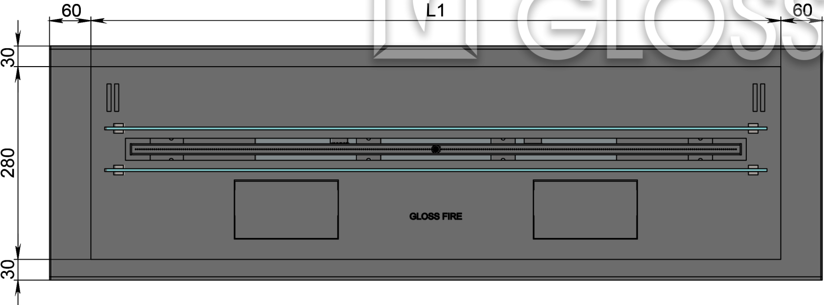
Вид сверху
