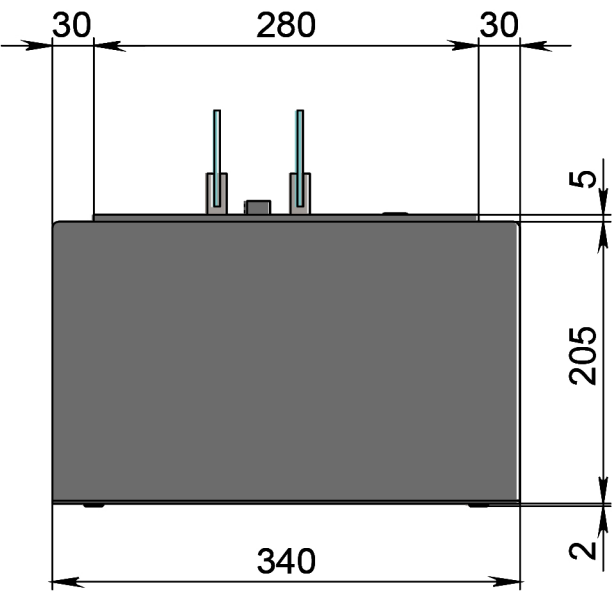
Вид сбоку
